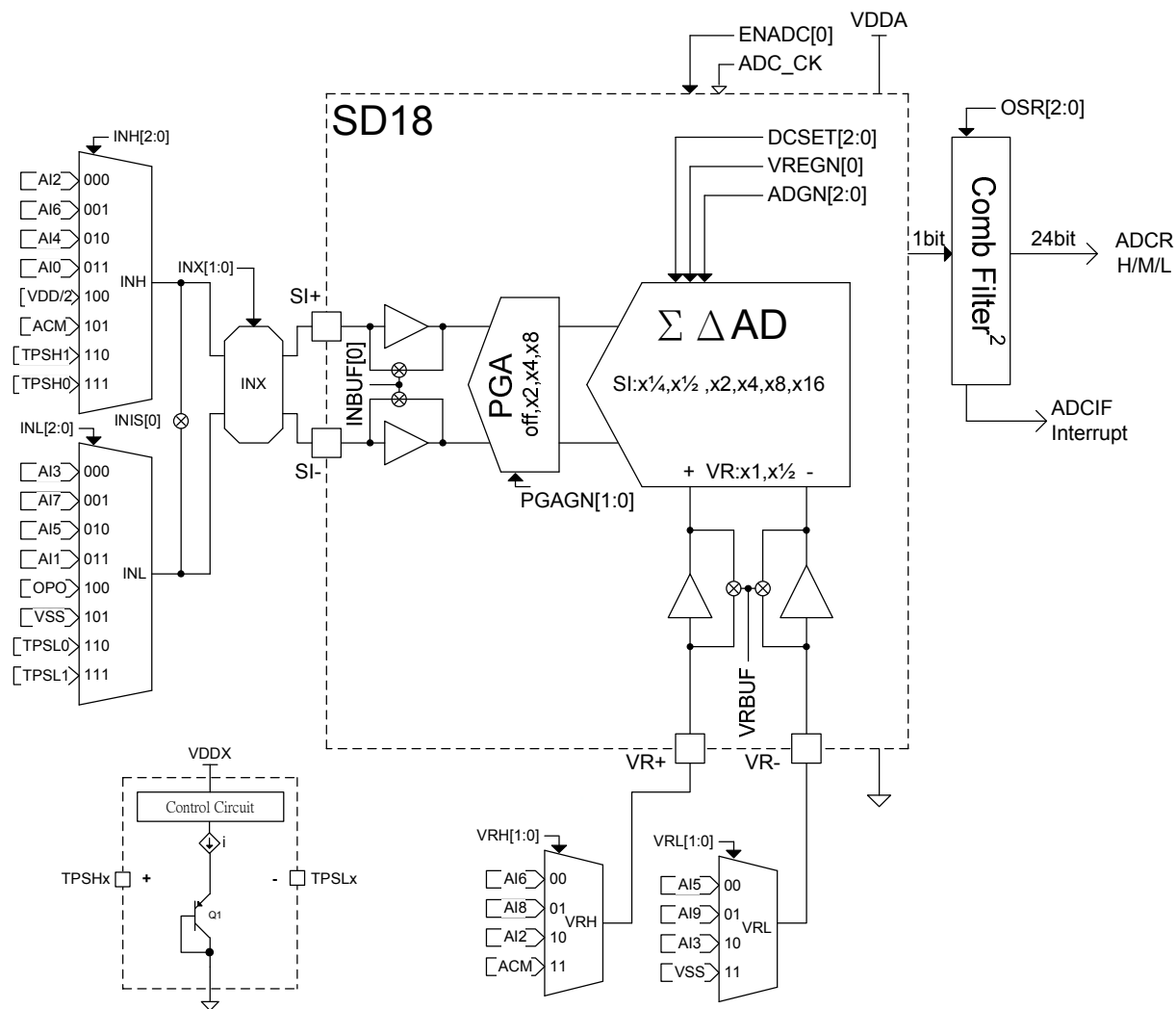
圖 4-2 SD18 Network
